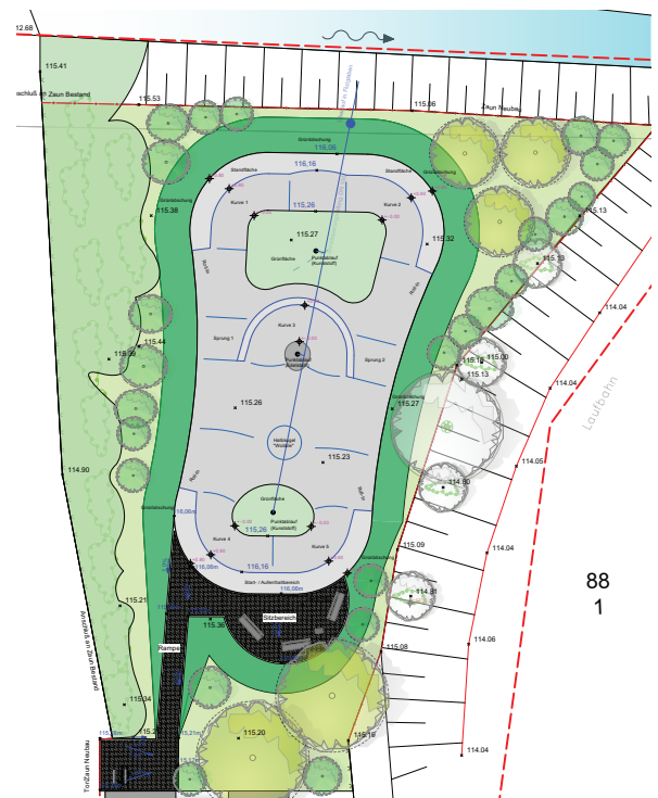
Lageplan
